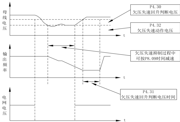
欠压失速抑制示意图
