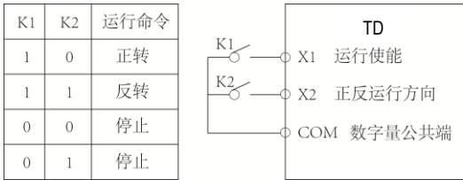
图 6-3 两线式模式 2
