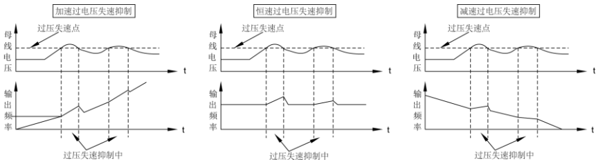
过压失速动作示意图
