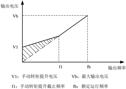
图 6-9 手动转矩提升示意图
