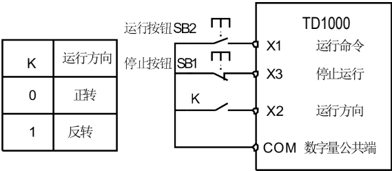
图 6-6 三线式模 2
