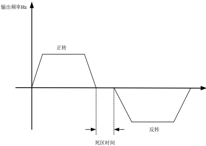
图 6-18 正反转死区时间示意图
